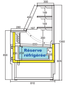
Version 2 étagères (3 éclairages)
