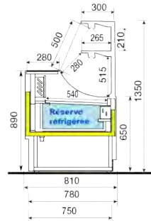
Version 1 étagère (2 éclairages)
